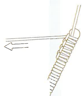
19. リーダーと本線となるPEラインを束ねる編み込みが完成
